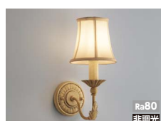
ERB6356X ¥25,500 LEDランプ×1 調 <100V> ● フロストクリプトン球40W形×1相当 消費電力：5.0W 39.0 lm/W(195 lm) 巾(170) 高(345) 出(229)mm 重:1.1kg
