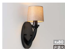
ERB6503U ¥23,500 LEDランプ×1 調 <100V> ● フロストクリプトン球40W形×1相当 消費電力：5.0W 39.0 lm/W(195 lm) 巾140 高334 出170mm 重:0.7kg
