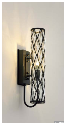
XRB1062X ¥59,500 LEDランプ×1 調 <100V> ● 透明シャンデリア球40W形×1相当 消費電力：5.0W 70.0 lm/W(350 lm) 巾(85) 高(457) 出(156)mm 重:2.2kg
