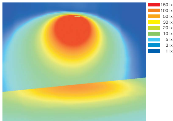
ERB6118W(RA-613LX1) 使用時 取付高さ：床より1.8m,首振り角度：壁側20°
