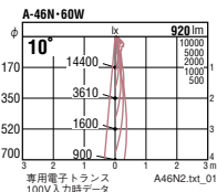
12Vφ50省電力ダイクロハロゲン球
